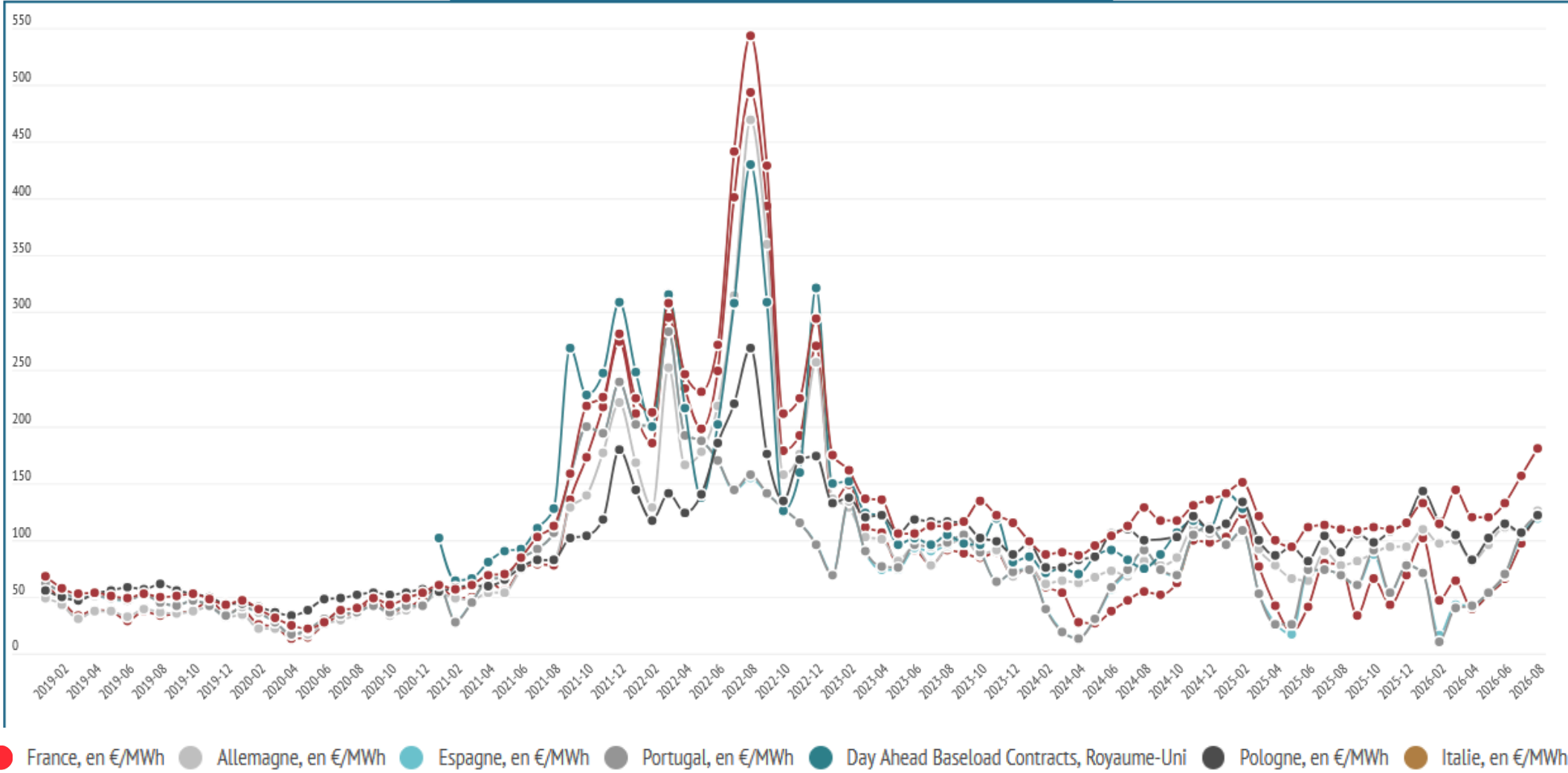
Prix de l'électricité sur le marché du gros - moyenne mensuelle. Source : Ember
